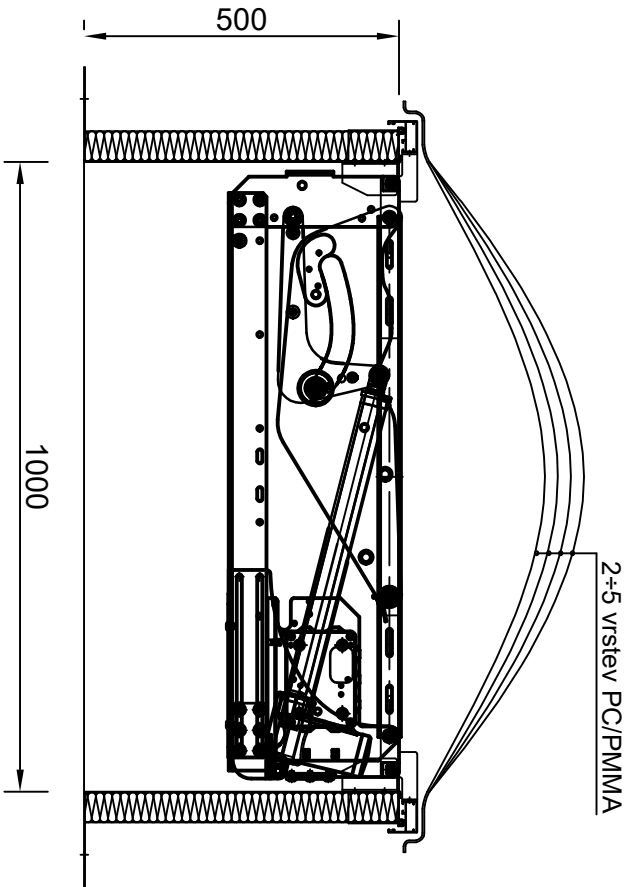
Podélný řez zavřený stav
