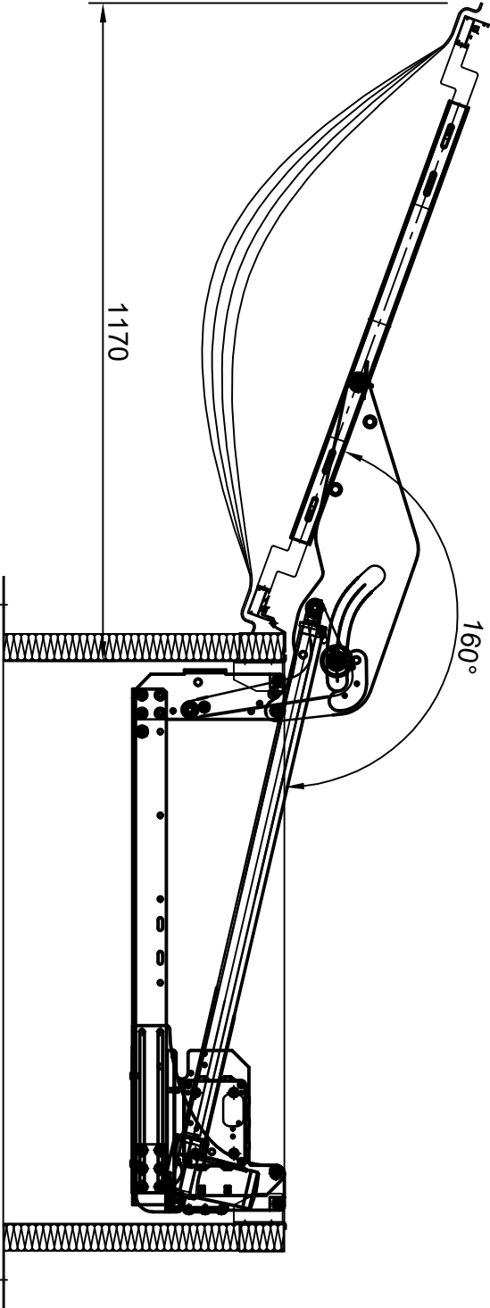
Detail manžety
